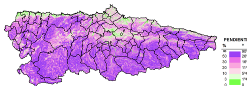
Superficie de Asturias según estratos de pendiente
