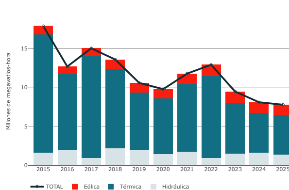
Producción anual de energía eléctrica según tipo
