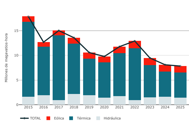
Producción anual de energía eléctrica según tipo
